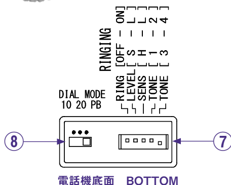
電話機底面 BOTTOM
